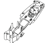
บังโคลนหลัง FENDER, REAR B7D-F1611-01
